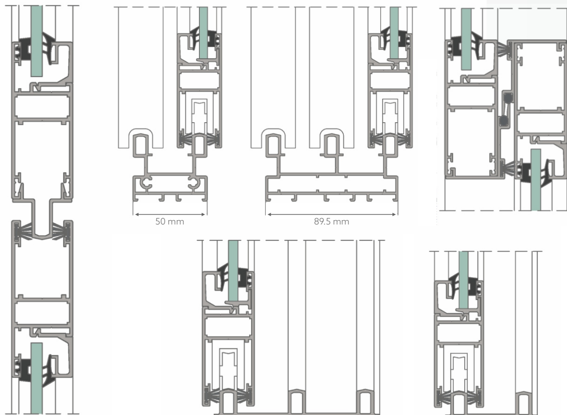
SECTION PAR PORTE COULISSANTE
