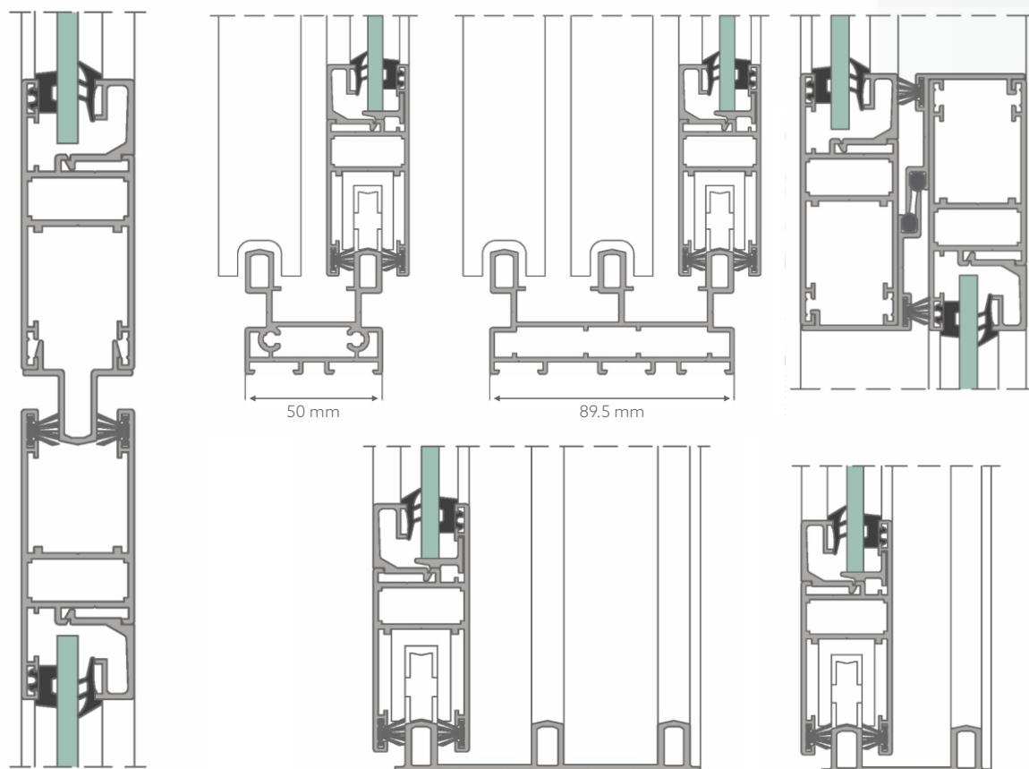
SECȚIUNE TRANSVERSALĂ PRIN CANATELE GLISANTE
