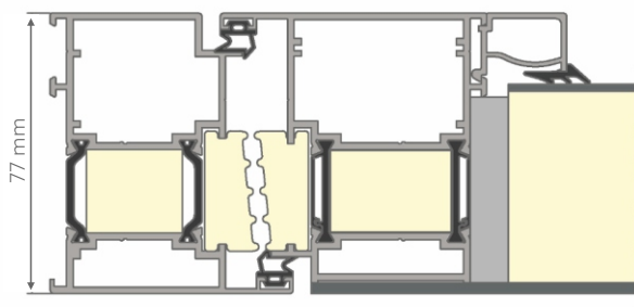
PORTE À PANNEAU MIS À NU DE 1 CÔTÉ OPTION AVEC LE JOINT D'ÉTANCHÉITÉ CENTRAL
