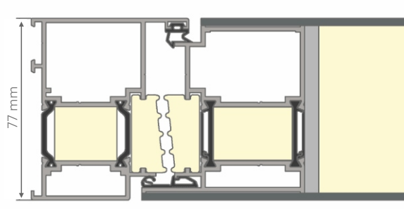
PORTE À PANNEAU MIS À NU DE 2 CÔTÉS OPTION AVEC LA MOUSSE ISOLANTE CENTRALE
