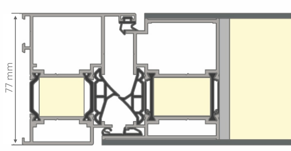
PORTE À PANNEAU MIS À NU DE 2 CÔTÉS OPTION AVEC LE JOINT D'ÉTANCHÉITÉ CENTRAL
