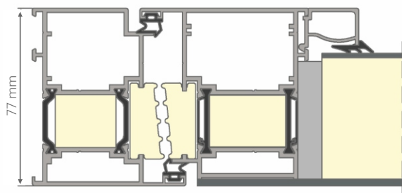
UȘĂ CU 1 PANOU PE ACELAȘI PLAN CU CADRUL, UNILATERAL VERSIUNEA CU GARNITURĂ CENTRALĂ
