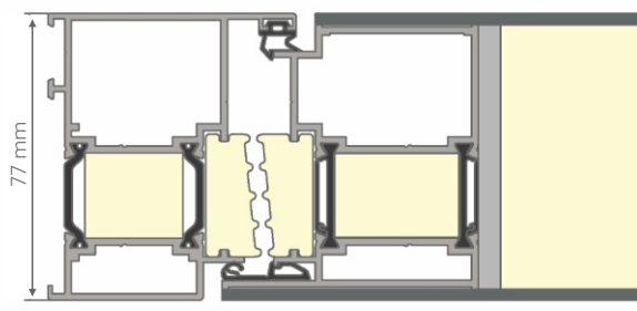
UȘĂ CU PANOU PE ACELAȘI PLAN CU CADRUL, DIN 2 PĂRȚI VERSIUNEA CU GARNITURĂ CENTRALĂ
